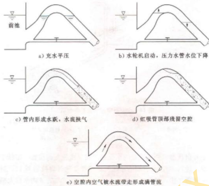
图 13 虹吸式进水口自动过程图
