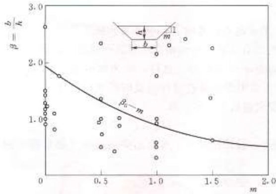
图2 \beta - m 关系曲线
