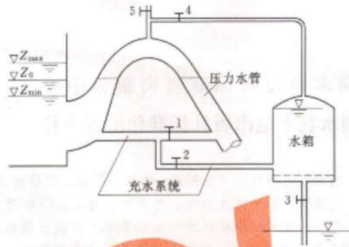
图 15 水箱式抽气系统图
