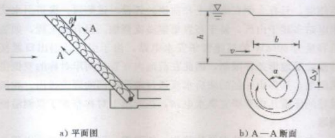
图1 涡管布置图
