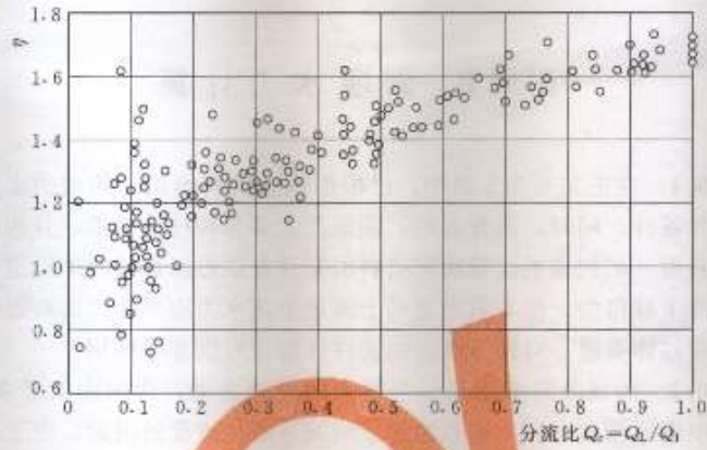
图6 \eta-Q 关系
