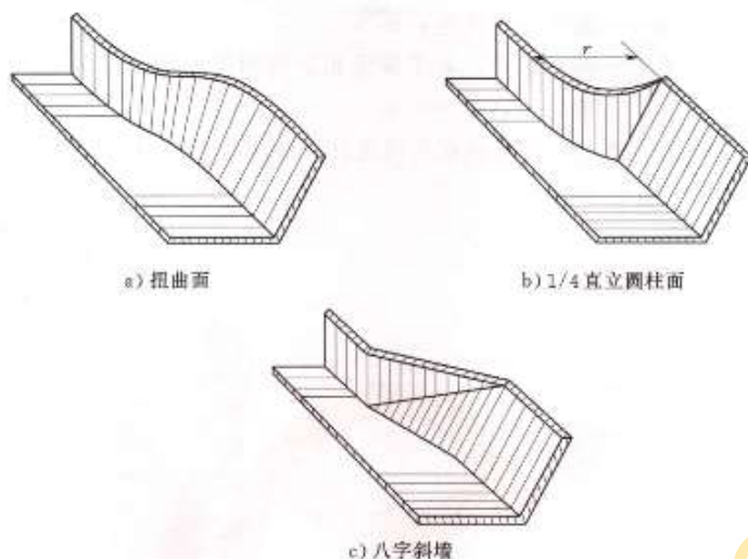
图 A.0.3-3 明渠渐变段形状图
