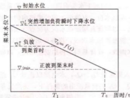
图 C.0.4-2 渠末水位随时间变化关系图
