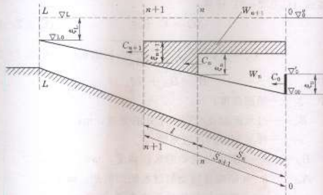
图 C.0.3-1 水电站突然丢弃负荷时涌波分析示意图
