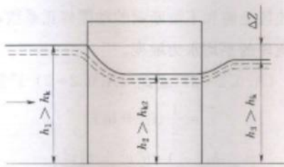
a) 水面线示意图
