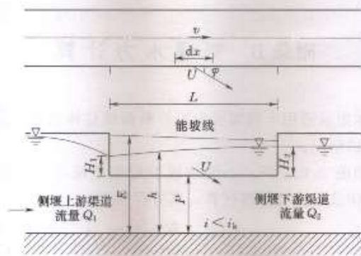
图 B.0.2 明渠侧堰溢流示意图
