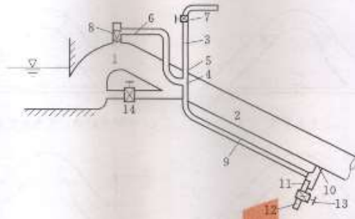
图 14 水力真空控制装置示意图
