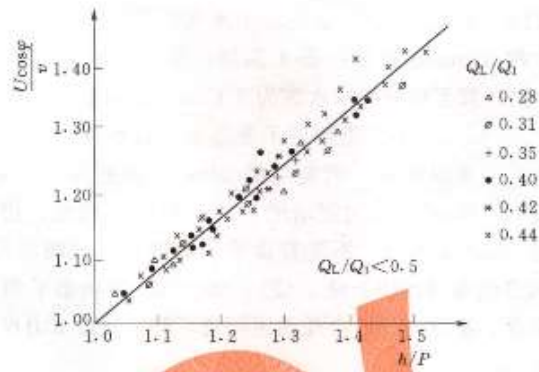
图8 U \cos \phi / v - h/P 关系
