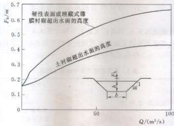
图3 美国垦务局渠道超高设计标准图
