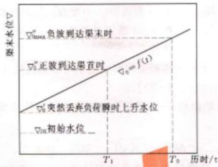
图 C.0.3-2 渠末水位随时间变化关系图
