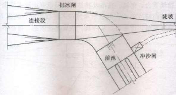
图 5 喀群一级水电站修改方案平面示意图
