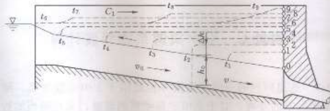
图 10 丢弃负荷后渠道内的非恒定流情况
