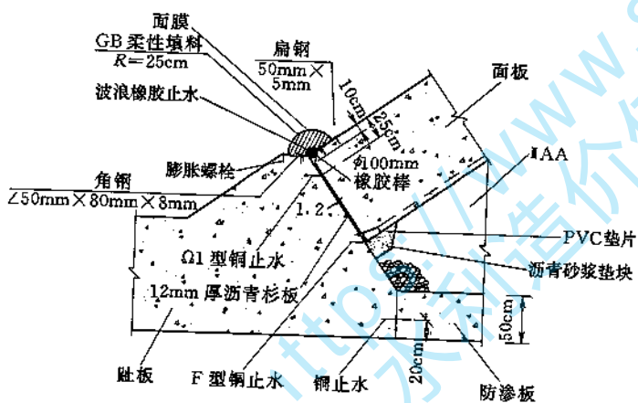
图10 水布垅面板堆石坝周边缝止水结构
