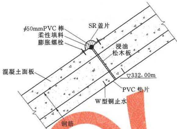
图8 水布锤面板堆石坝永久水平缝止水结构示意图
