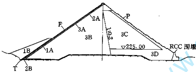
图 1 水布垭面板堆石坝断面分区图
