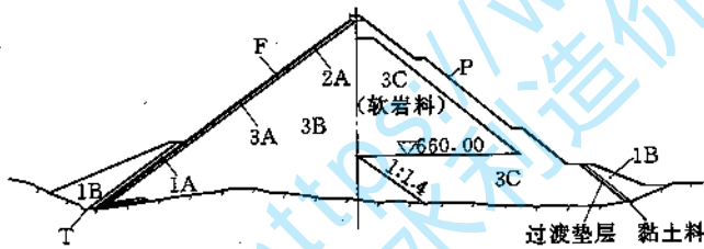
图5 天生桥一级面板堆石坝断面分区图
