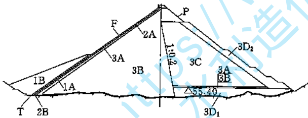
图 2 巴贡面板堆石坝断面分区图
