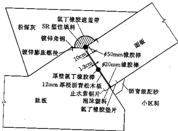
图9 滩坑面板堆石坝周边缝止水结构
