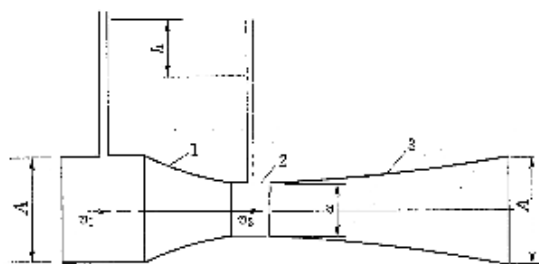
1—收缩管；2—喉管；3—扩大管
