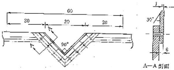
图 1 复式堰构造和尺寸 (单位: mm)
