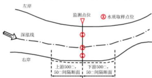
图 6 大河监测河段的监测断面布置示意图
