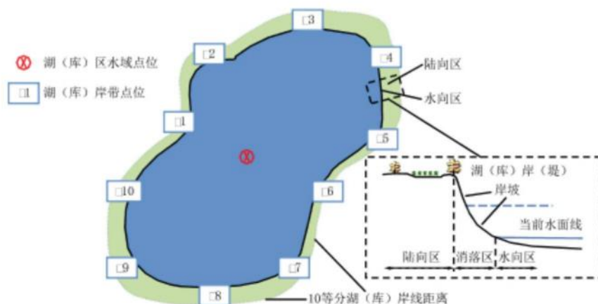
图7 湖(库)监测点位布置示意图
