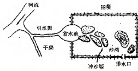
图2 引水拉沙工程部署示意图
